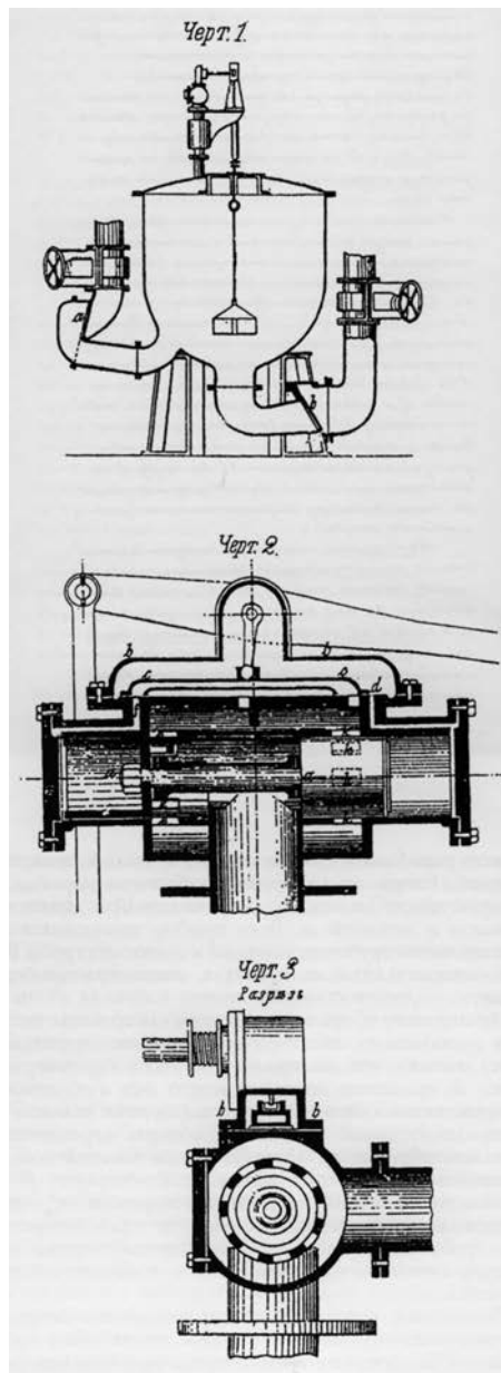
Ежектор Шона
