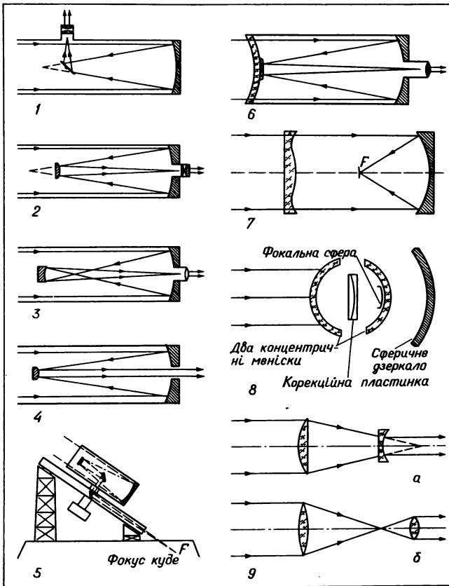
Мал. 24. Лінзові (а, б) та дзеркальні (1 — 8) оптичні системи телескопів: а — Галілея, б — Кеплера, 1 — Ньютона, 2 — Кассегрена, 3 — Грегори, 4 — Мерсенна, 5 — куде, 6 — Максутова, 7 — Шмідта, 8 — система супершмідт
