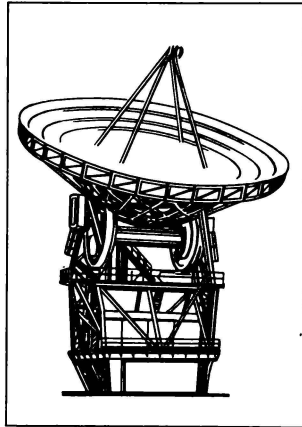
Мал. 31. 22-метровий прецизійний радіотелескоп Фізичного інституту АН СРСР ім. П. М. Лебедева
