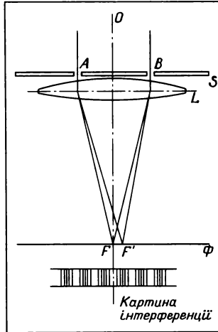
Мал. 16. Схема утворення інтерференційної картини
