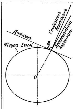
Мал. 6. Астрономічна та геодезична вертикалі
