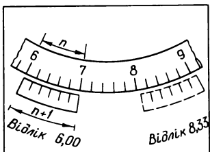
Мал. 5. Принцип роботи з верньєром
