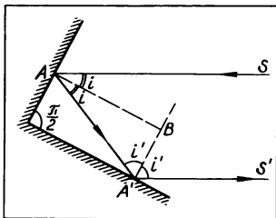
Мал. 9. Хід падаючого S і відбитого S' променя у кутниковому відбивачеві
