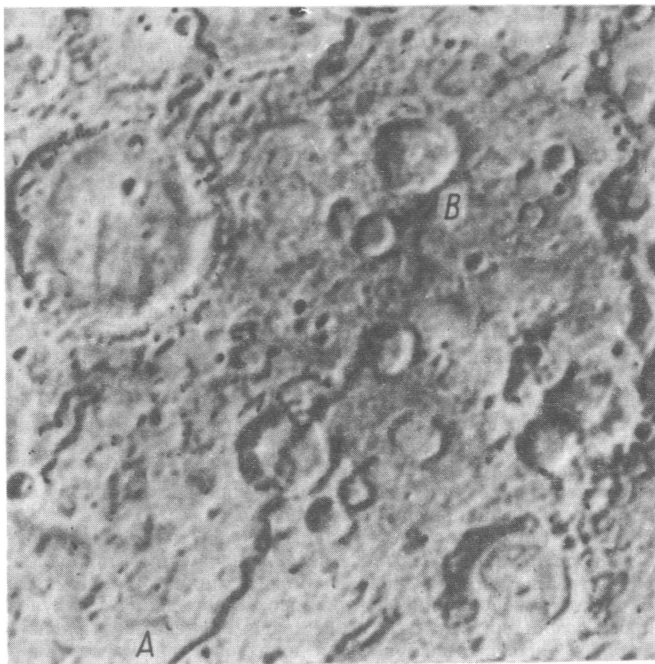
Мал. 15. Ескарп AB на поверхні Меркурія. Його довжина (на фотознімку видно лише його частину) досягає 500 км (фотознімок з космічного апарата «Маріонер-10»)
