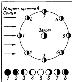
Мал. 38. Фази Місяця: 1 — новий місяць, 3 — перша чверть. 5 — повня (повний місяць), 7 — третя (остання) чверть
