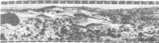
Мал. 17. Панорама Марса, передана 3.08.1976 р. з поверхні Марса «Вікінгом-1». Ліворуч — кам'яна брила Великий Джо (1×3 м), видно піщані дюни
