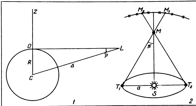
Мал. 25. Горизонтальний добовий ( p ) і річний ( \pi ) паралакси, визначення яких дає змогу встановити відстані відповідно до об'єктів Сонячної системи (1) та близьких зір (2)
