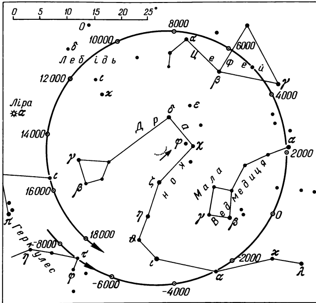
Мал. 30. Прецесійний рух Північного полюса світу (точками в центрі показано рух полюса екліптики)
