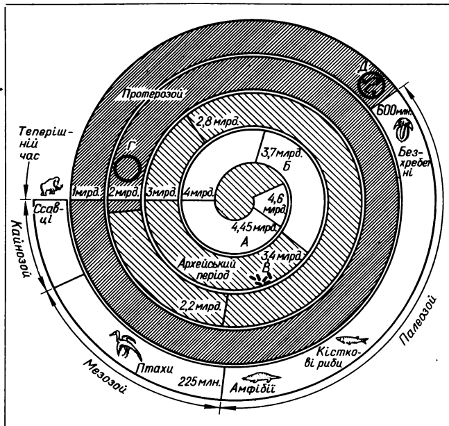
Мал. 13. Спиральний годинник еволюції Землі. Літерами позначено час виникнення найстаріших місячних (А) і земних (В) порід, найперших викопних клітин (В), решток фотосинтезуючих рослин (Г) і докембрійських безхребетних (Д).
