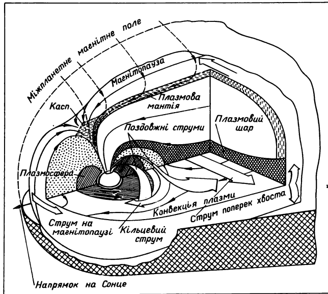
Мал. 21. Будова земної магнітосфери
