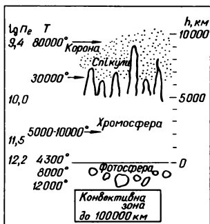
Мал. 34. Схема будови атмосфери Сонця; вказано температури і концентрації електронів залежно від висоти
