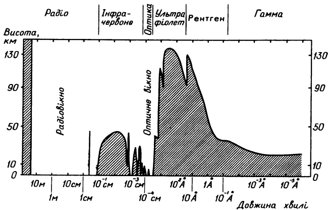
Мал. 10. Поглинання випромінювання у земній атмосфері. Крива відповідає висоті, на якій поглинається 50 % випромінювання
