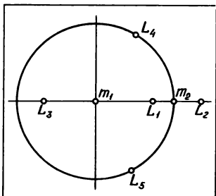
Мал. 20. Лібраційні точки у задачі трьох тіл: двох великої маси m_1 та m_2 і тіла L малої маси. L_4 , L_5 — трикутні лібраційні точки, L_1 , L_2 , L_3 — колінеарні
