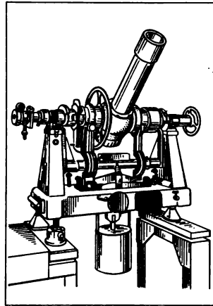
Мал. 27. Пасажний інструмент
