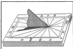
Мал. 35. Горизонтальний сонячний годинник
