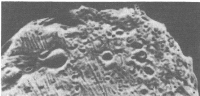
Мал. 37. Супутник Марса Фобос зблизка. Видно смуги — тріщини, пов'язані спільністю походження з великим кратером Стікні
