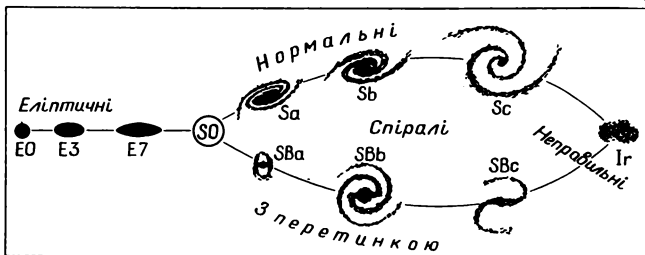
Мал. 39. Хабблівська класифікація галактик
