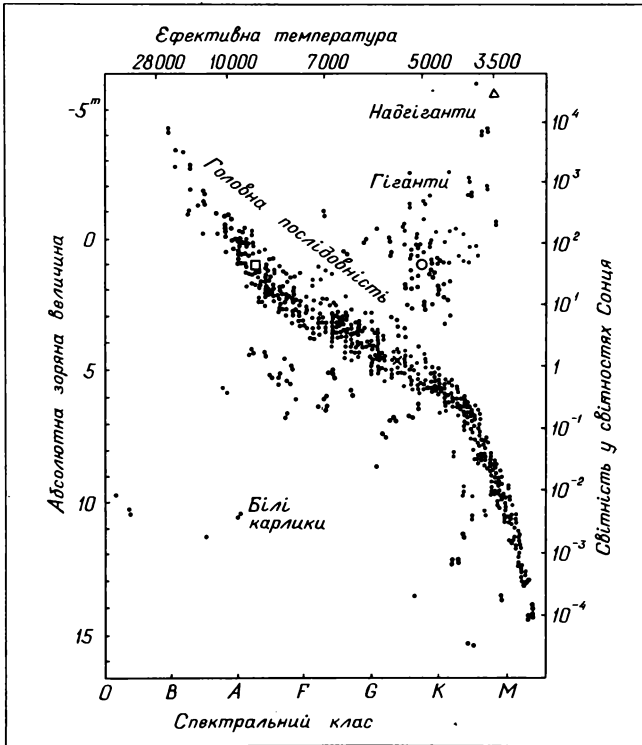
Мал. 11. Діаграма Герцшпрунга — Ресселла
