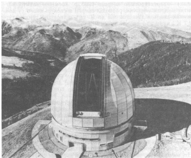
Мал. 32. Найбільший у світі рефлектор Спеціальної астрофізичної обсерваторії АН СРСР (у горах Кавказу поблизу станції Зеленчуцької). Діаметр дзеркала 6 м
