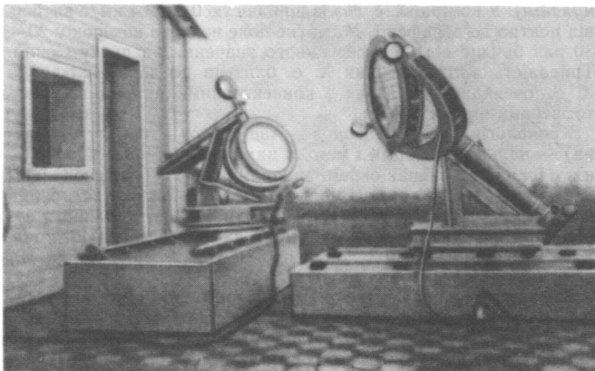
Мал. 40. Целостат горизонтального сонячного телескопа
