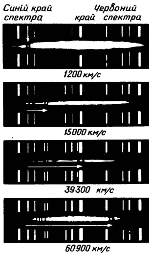
Мал. 41. Червоне зміщення в спектрах галактик
