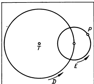
Мал. 14. Епіцикл E — допоміжне коло, яким у системі Птолемея рухається планета P і центр якого в свою чергу рухається навколо Землі T
