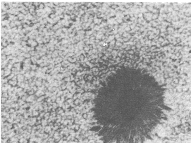
Мал. 36. Велика сонячна пляма на фоні грануляційної картини (фотознімок зроблений з борта ШСЗ)
