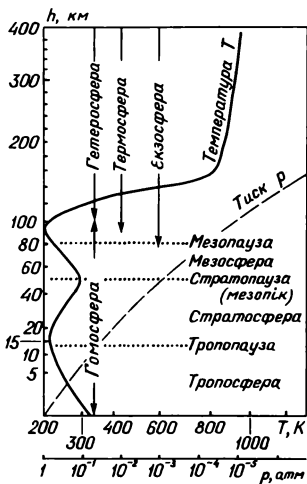
Мал. 3. Будова атмосфери Землі
