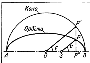
Мал. 1. Справжня \nu та ексцентрична E аномалії
