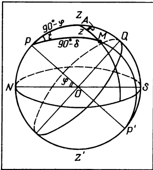
Мал. 26. Паралактичний трикутник
