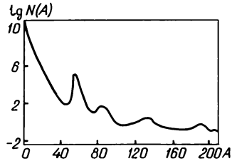
Мал. 29. Відносна поширеність хімічних елементів у Всесвіті
