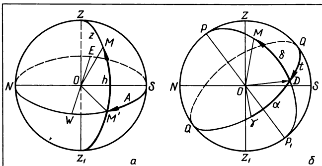
Мал. 33. Горизонтальна (а) і екваторіальна (б) системи небесних координат
