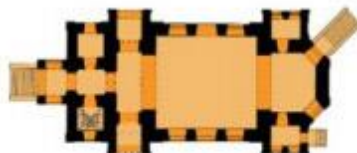
Схема плану Покровської церкви у с. Рубанівське. Креслення автора, 2008 р.
