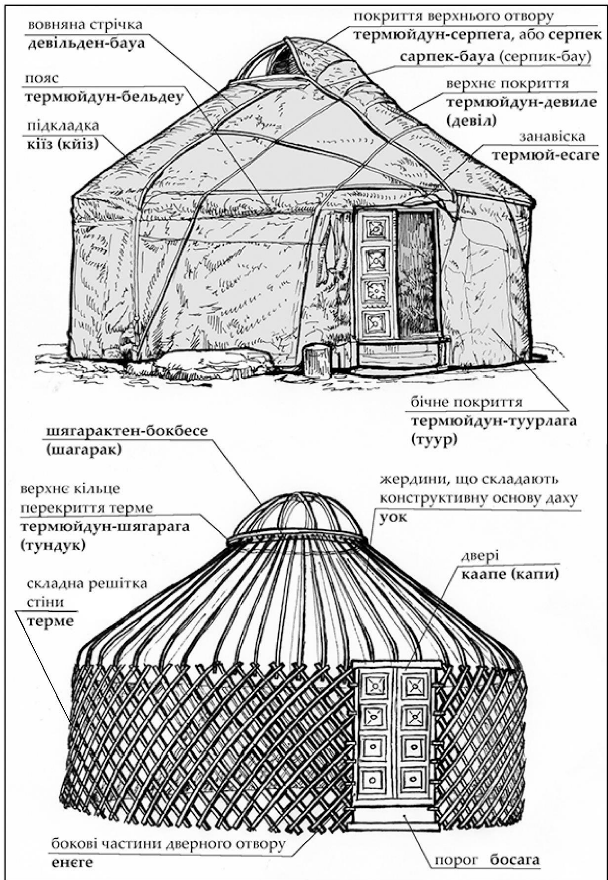
Рис. 3. Основні деталі ногайської юрти терме (назви складових за А. Архиповим та Б. Кочекаєвим). Малюнок автора (2020 р.).
