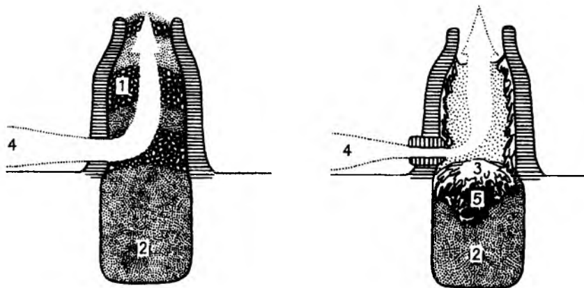
Технологія виплавки заліза у сиродутному горні (реконструкція): 1) залізна руда 2) деревне вугілля 3) нагнітання повітря 4) залізна криця (Schlette 1979)
