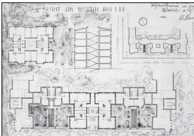
Рисунок 3. Проект будинку. Поповерхові плани, розріз. 1934 р.
