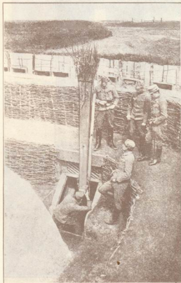
Періскоп, прилад до обсервації передпілля зі земляном.
