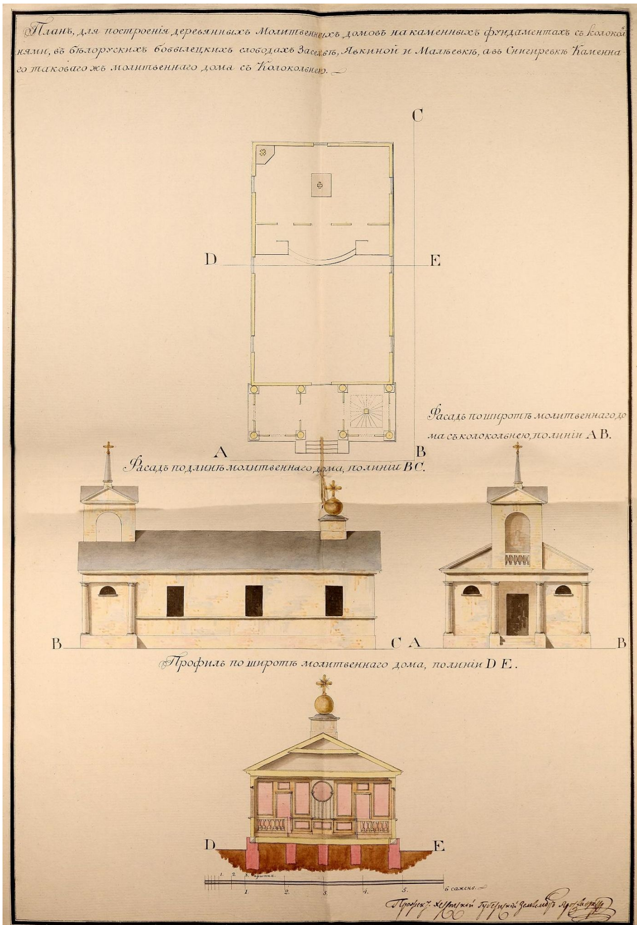
Креслення будівлі молитовного будинку, виконане херсонським губернським землеміром Ярославським (1816) ДАОО. – Ф. 1, – Оп. 220. – Спр. 2. – Ч. 2. – 1814 р. – Арк. 109а
