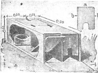
Рис. 179. Самозамикаюче гніздо для несучок. Передня стіна рухома тільки до середини, так, що курка не може сама вийти. В горішній стіні зарисований отвір, куди курки вилітає. Для догідности можна робити подвійні гнізда, як се подано на рисунку.
