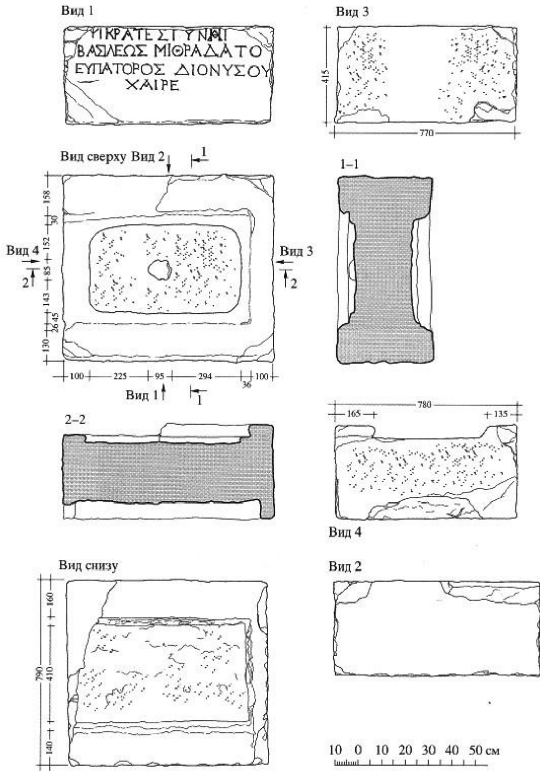
Креслення постаменту Гіпсікратії. Фанагорія, Російська Федерація
