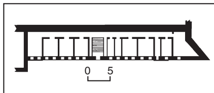
489.1.35. Набиральня та коректорська. 489.1.35. План першого поверху.
