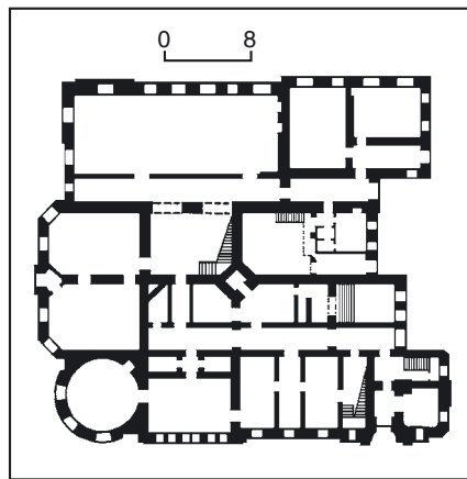
521.16. План першого поверху. 521.16. Вул. Л. Толстого, 7/2. Особняк.
