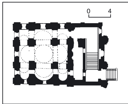
489.1.54. План.
