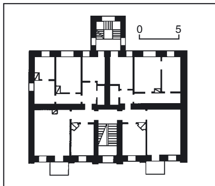
541.6. План другого поверху.
