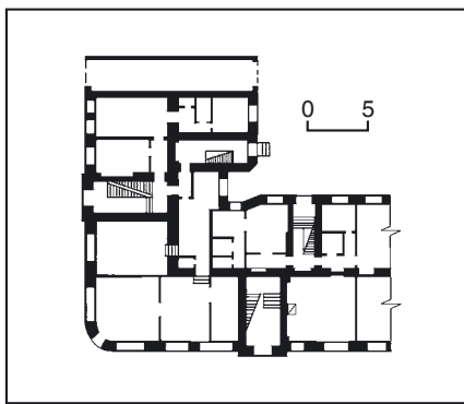
496.11. Вул. Січневого повстання, 18/29. 496.11. План першого поверху.
