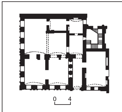
489.1.24. План другого поверху.
