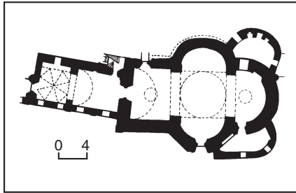
489.2.31. План.
