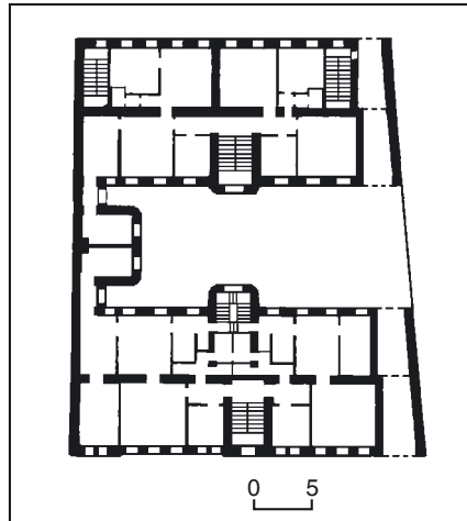
514.13. План першого поверху.
