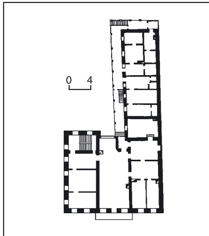
498.2. Вул. Г. Сковороди, 5-а. 498.2. План другого поверху.
