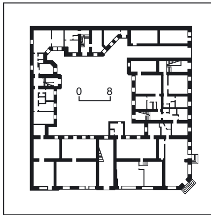
541.15. План першого поверху.
