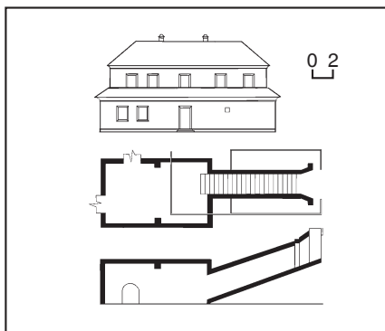
489.1.41. План споруди № 9.
