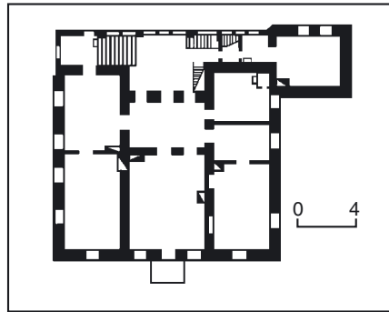
542.4. Вул. Хорива, 16/7. 542.4. План другого поверху.
