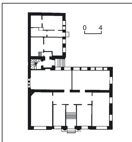
506.1. Вул. Спаська, 12. 506.1. План першого поверху.
