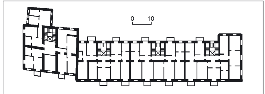
544.21. План четвертого поверху.
