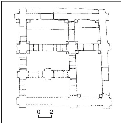
489.1.55. План церкви (трапезної).
