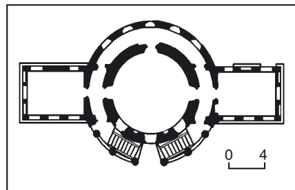
532.7. План
