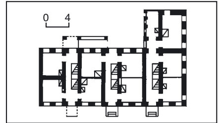
532.16. Келії. Корпус № 9. 532.16. План першого поверху.
