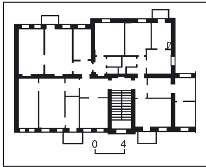
576.7. План третього поверху.
