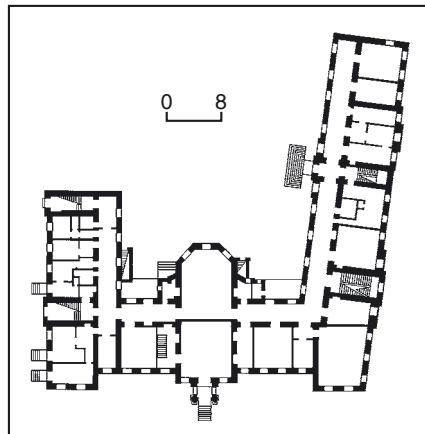
489.5.4. План першого поверху.
