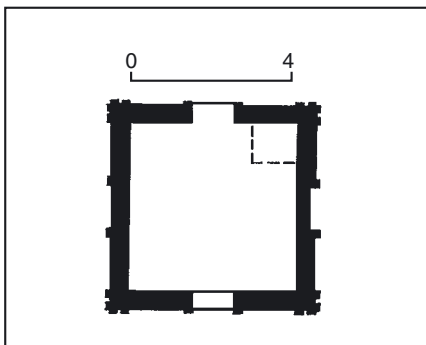
489.2.30. План. 489.2.30. Сторожка.
