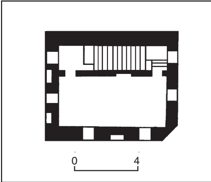
489.1.23. План другого поверху.
