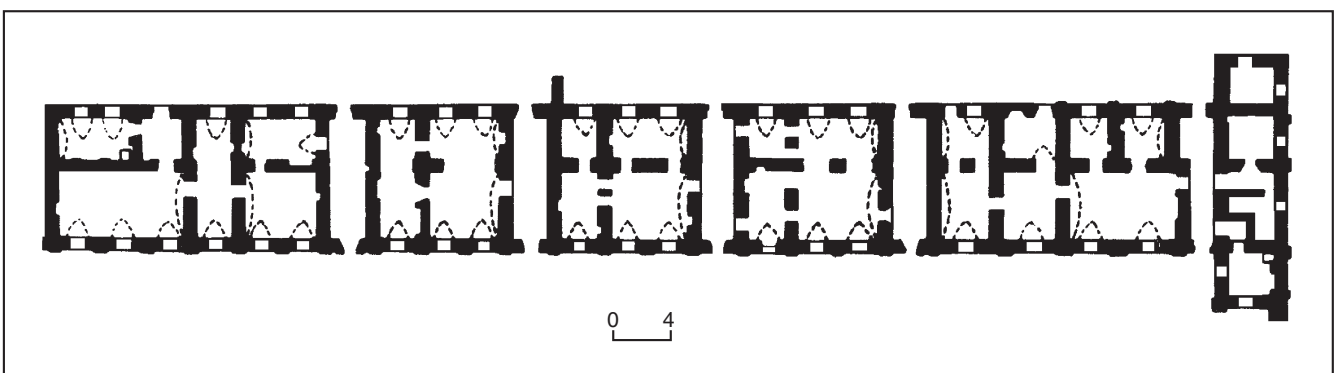
489.1.18. План першого поверху.
