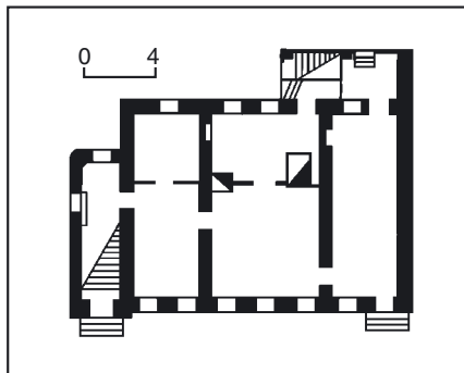
542.7. План першого поверху.
