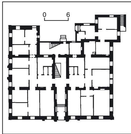
534.11. План першого поверху. 534.11. Вул. І. Франка, 33.
