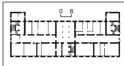
563.1. План другого поверху. 563.1. Бульв. Т. Шевченка, 27.
