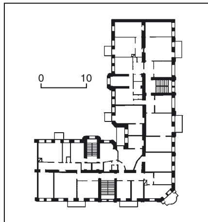
542.5. План другого поверху. 542.5. Вул. Хорива, 21—23.
