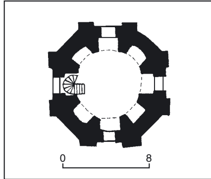
489.5.1. План другого ярусу.
