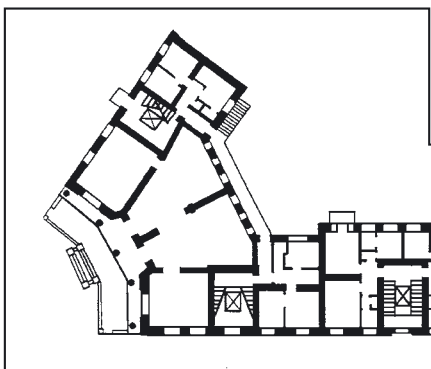
521.13. План другого поверху.
