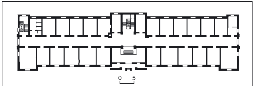
495.7. План першого поверху.
