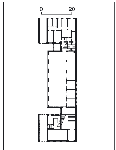
544.19. План першого поверху.
