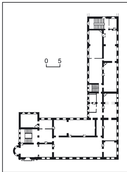
541.24. План другого поверху. 541.24. Вул. Б. Хмельницького, 11.
