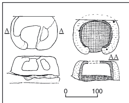
517. План та розріз печі будівлі № 1.
