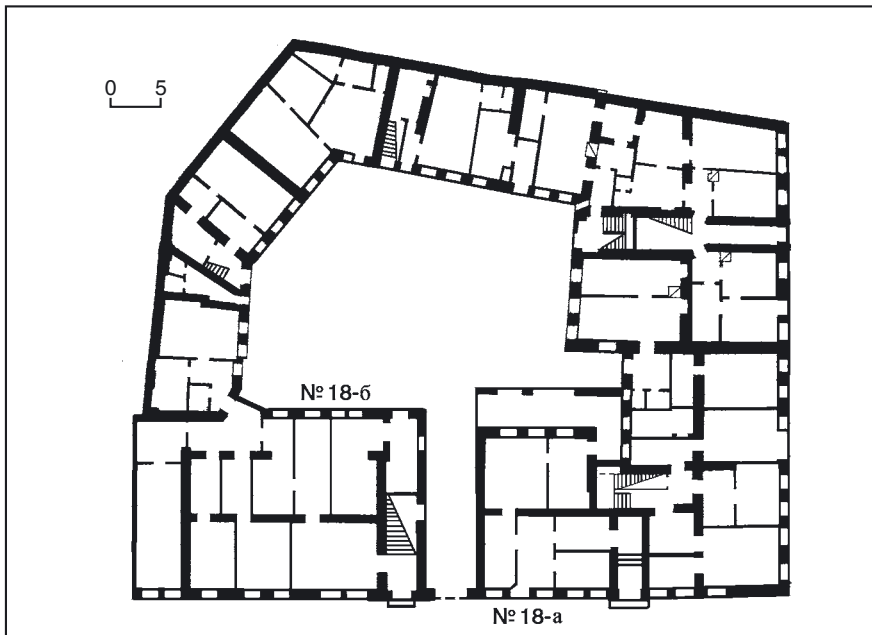
542.11. Вул. Хорива, 18/10, 18-а, 18-б. План першого поверху.
