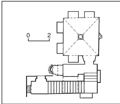
489.1.41. План споруди № 3.
