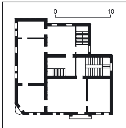
563.23. План другого поверху.
