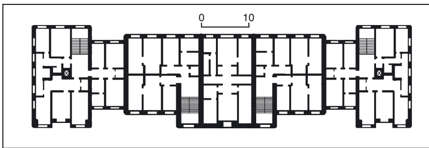
544.20. План дев'ятого поверху. 544.20. Вул. Хрещатик, 25.
