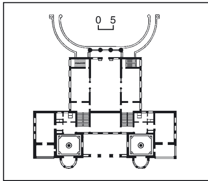
496.7. План першого поверху.
