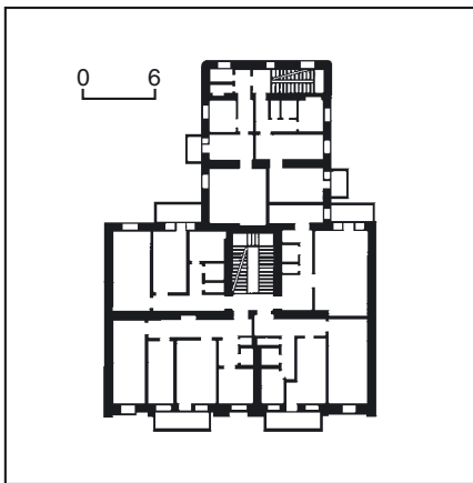
561.15. План другого поверху. 561.15. Вул. Червоноармійська, 41.
