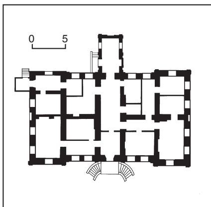
489.1.19. План.
