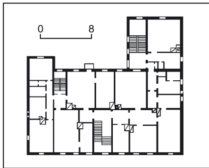
502.7. Вул. Софійська, 23. 502.7. План другого поверху.
