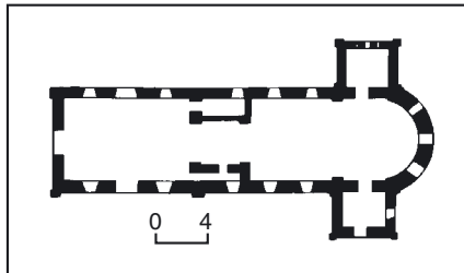
489.4.41. План.
