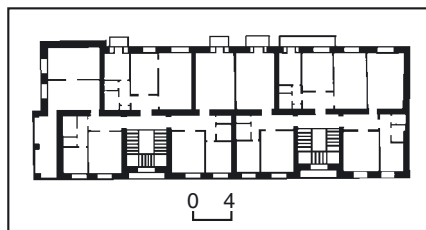
559.1. План другого поверху. 559.1. Вул. Чапаєва, 3.
