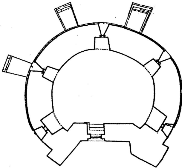
Башта Нова, XVI ст. План першого ярусу. Обміри автора
