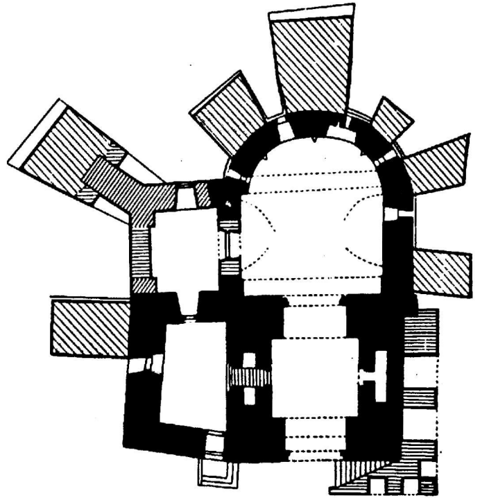
“Вежа Мурована”. План першого ярусу із зазначенням первісного ядра. Обміри автора
