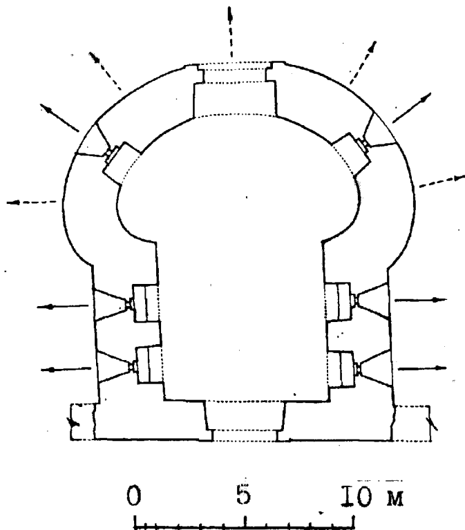
Луцька брама, XV—XVI ст. План першого ярусу. Обміри автора
