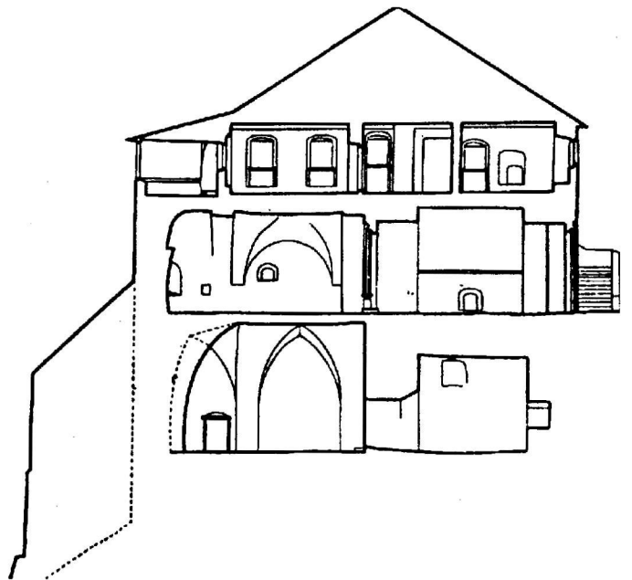
“Вежа Мурована”. Поперечний переріз. Обміри автора
