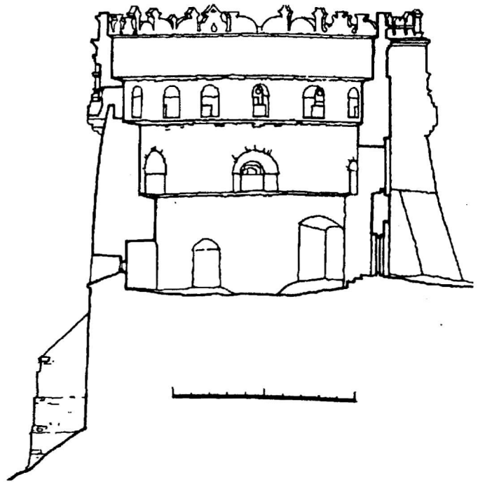
Башта Нова, XVI ст. Поперечний перекрій. Обміри автора
