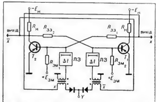
Схема імпульсно-потенціального тригера з лічбовим входом.
