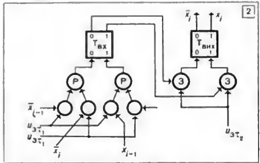
1. Блок-схема регістра в імпульсно-потенціальній елементній структурі зі зсувом управо: u_{пi} — керуючий потенціал передавання на регістр слова x_1, x_2, x_3, x_4 ; З — імпульсно-потенціальний збіг; Р — імпульсний розподіл сигналів; u_3 — керуючий сигнал зсуву 2. Блок-схема розряду регістра в потенціальній елементній структурі: u_{3т1}, u_{3т2} — сигнали, які керують зсувом.
