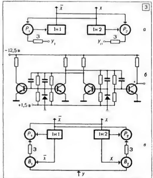
1. Потенціальні схеми: а — збігу; б — розділення. 2. Потенціально-імпульсні вентилі: а — принципова схема з вхідним потенціальним сигналом від підсилювача на трансформаторі; б — блок-схема групи вентилів з вихідним формувачем Ф. 3. Схеми тригера: а — блок-схема; б — принципова схема на напівпровідникових елементах з вихідним підсилювачем; в — блок-схема тригера в лічильному режимі.
