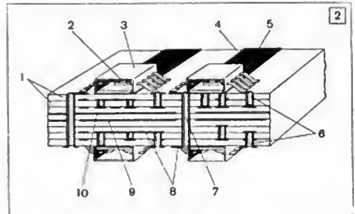
1. Типові електричні схеми інтегральних логічних елементів на біполярних транзисторах. 2. Структура багатошарової друкованої плати для монтажу інтегральних схем: 1 — шари з епоксидного склопластику; 2 — активний елемент; 3 — інтегральна схема; 4 — тепловідвідні смужки; 5 — контактні циліндри; 6 — мікшарові з'єднання; 7 — свід; 8 — шари друкованого монтажу; 9 — шини живлення; 10 — заземлення.
