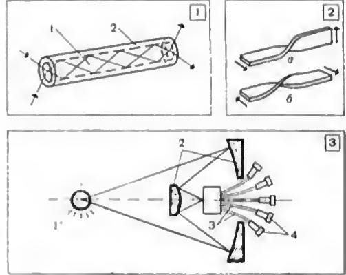
1. Окреме волокно: 1 — сердечина, 2 — оболонка. 2. Поворотник зображення: а — на 90°, б — на 180°. 3. Схема волоконного дисектора зображення: 1 — джерело світла; 2 — опукле та угнуте дзеркала; 3 — елементи волоконного джгуту; 4 — приймачі зображення.
