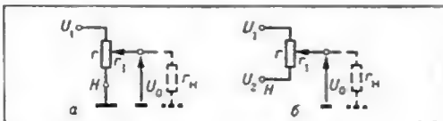
Схеми вимірювання подільника напруги.
