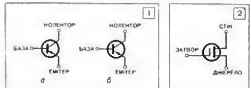
1. Схеми напівпровідникових тріодів: а — n-p-n -типу; б — p-n-p -типу.
