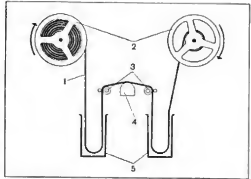
Схема стрічкопротяжного механізму.
