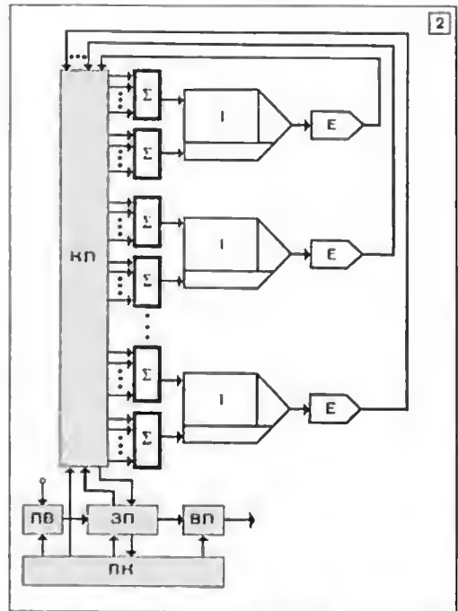
1. Схема узагальненого інтегратора: \Sigma — суматор пристроїв; І — інтегратор; Е — екстраполатор. 2. Структура цифрової інтегрувальної машини.
