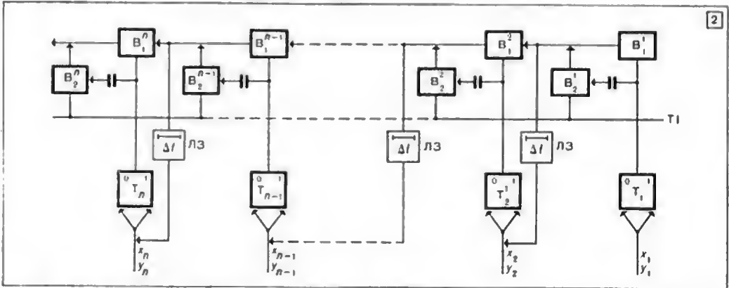
1. Схема нагромаджувального суматора з послідовним переносом. 2. Схема нагромаджувального суматора з паралельним переносом.
