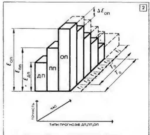
1. Типологія прогнозів. 2. Побудова системи взаємного прогнозування.
