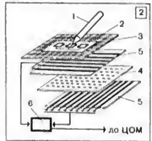
1. Безконтактна (фотоелектрична) клавіатура: 1 — клавіша; 2 — важіль з прорізами; 3 — блок джерел світла; 4 — світлові промені (проходять через прорізи і затримуються виступами важеля); 5 — блок фотоелементів. 2. Панель графічного введення з контактним олівцем: 1 — олівець або кулькова ручка; 2 — ескіз; 3 — аркуш поліхлорвінілу з сіткою ліній, відповідних провідникам; 4 — панель (46 см × 61 см) із скловолокна завтовшки 0,1 мм а нанесеними через 5 мм провідниками; 5 — тонка поліефірна плівка з отворами в місцях перетину провідників; 6 — пристрій вироблення цифрових значень координат.
