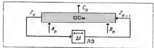
Функціональна схема послідовного суматора.
