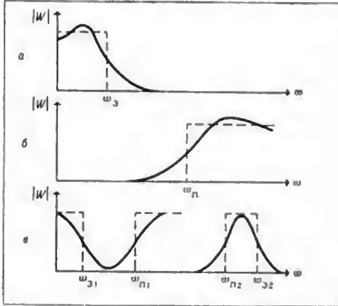
Частотні характеристики фільтрів: а — низьких частот; б — високих частот; а — запираючого і лузко-смугового.
