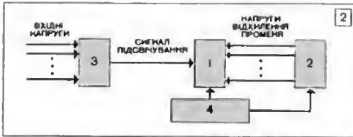
1. Блок-схема електроннопроменевого індикатора статичного типу. 2. Блок-схема електроннопроменевого індикатора динамічного типу.
