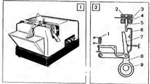
1. Перфоратор стрічковий типу ПЛІ-80. 2. Механізм набірника коду й пробивання стрічкового перфоратора: 1 — кодовий електромагніт; 2 — матриця; 3 — перфорстрічка; 4 — рама; 5 — пуансон; 6 — зворотна рама; 7 — штовхач; 8 — шатуни; 9 — ексцентрикний вал.
