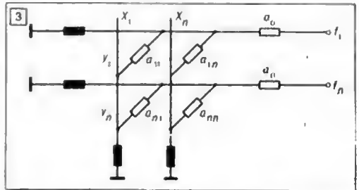
1. Електрична схема методу нульових власних провідностей. 2. Схема лямбда-аналогової моделі системи алгебричних рівнянь. 3. Схема дзета-аналогової моделі системи алгебричних рівнянь.
