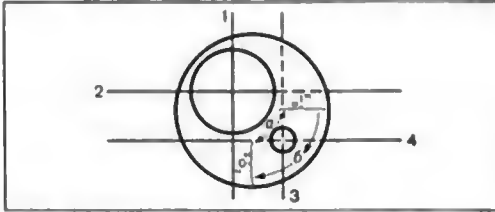
Схема трансфлюксора.
