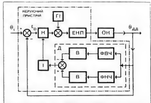
Функціональна схема самонастроюваної параметричної системи: ФВЧ — фільтр високих частот; ФНЧ — фільтр низьких частот; В — випрямляч.
