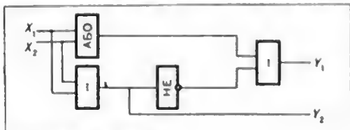
Блок-схема Півсуматора.
