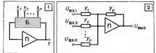
1. Блок-схема операційного підсилювача.
