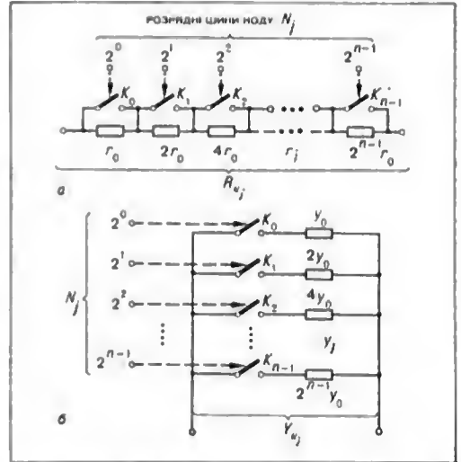
Схема кола постійних резисторів: а — ввімкнених послідовно, б — ввімкнених паралельно.
