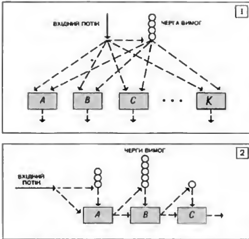
1. Схема багатолінійної системи масового обслуговування. 2. Схема багатофазної системи масового обслуговування. 3. Схема мережі масового обслуговування.
