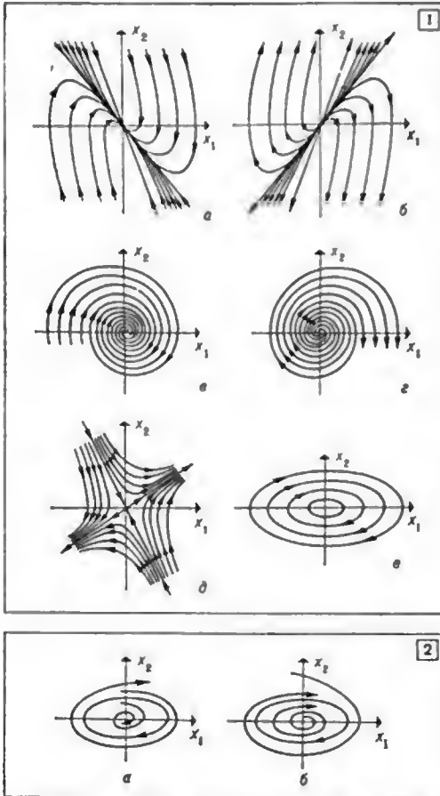
1. Типи особливих точок: а — стійкий вузол; б — нестійкий вузол; в — стійкий фокус; г — нестійкий фокус; д — сірло; е — центр. 2. Граничні цикли: а — нестійкий; б — стійкий.
