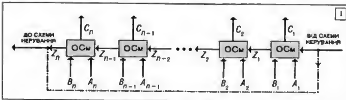
1. Функціональна схема паралельного суматора. 2. Схема формування переносу в паралельному суматорі.
