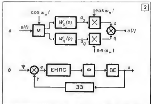
1. Система керування на змінному струмі: а — блок-схема; б, в — форми сигналів несучої частоти; з — форма сигналів, модульованих за амплітудою. 2. Еквівалентні блок-схеми: а — пристрою з амплітудною модуляцією; б — системи керування на змінному струмі.
