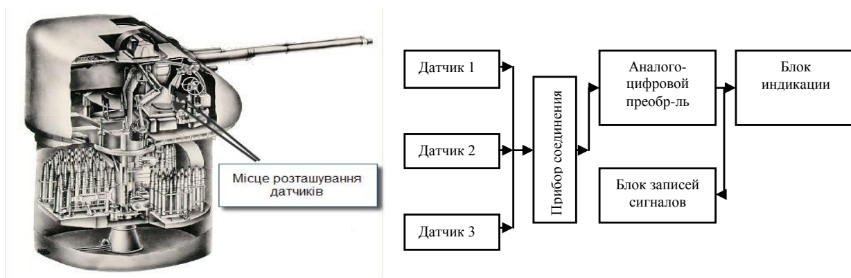
Рис. 1. Структура измерительной установки с местами расположения датчиков в КАУ АК-176
