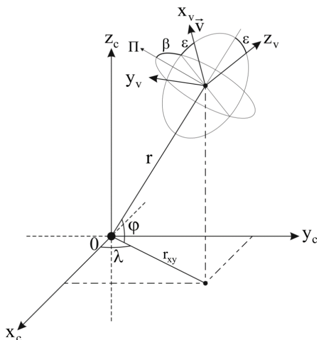
Рис. 2. Зв'язана "швидкісна" система координат
