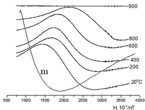
Рис. 2. Спектри феромагнітного резонансу природного магнетиту (m) і зразків магеміту прогрітих за вказаних температурах
