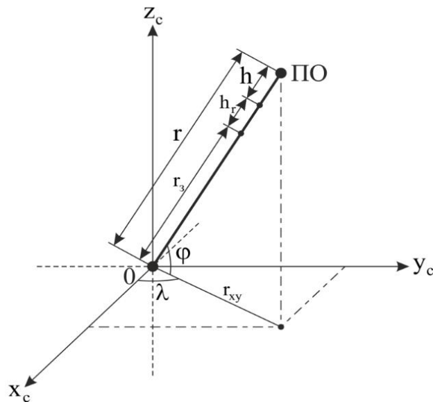
Рис. 1. Географічна та "світова" системи координат
