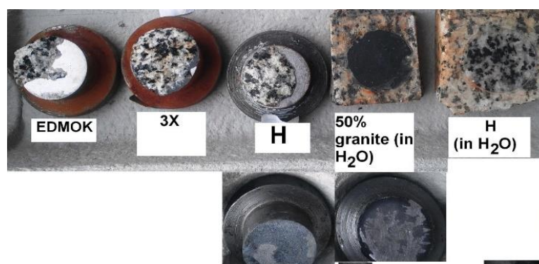
Рис. 1. Вид адгезионных соединений после отрыва, с применением составов ЭДМОК, 3X и H (незаполненный). Остатки гранита на склейках – у образцов в нормальных условиях; склейки на граните – от образцов после 10 дней выдержки в воде. Внизу – вид адгезива на стальной поверхности
