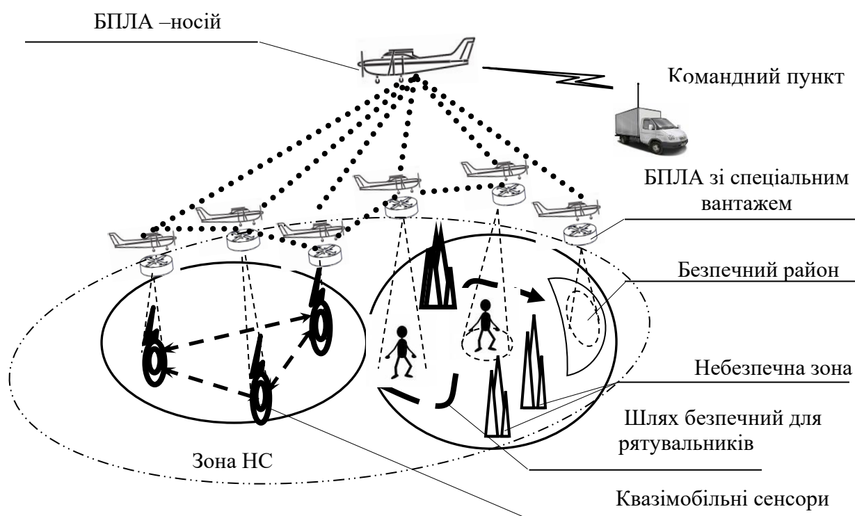
Рис. 5. Приклад застосування «літаючих сенсорних мереж» для проведення пошуково-рятувальних робіт в зоні надзвичайної ситуації
