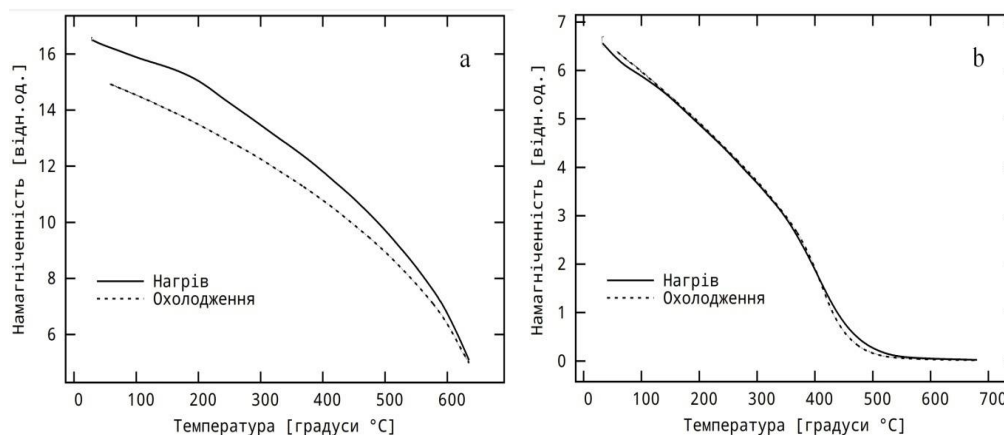
Рис. 1. Термомагнітні криві зразків прогрітих при 300 (a) і 700 °C (b)
