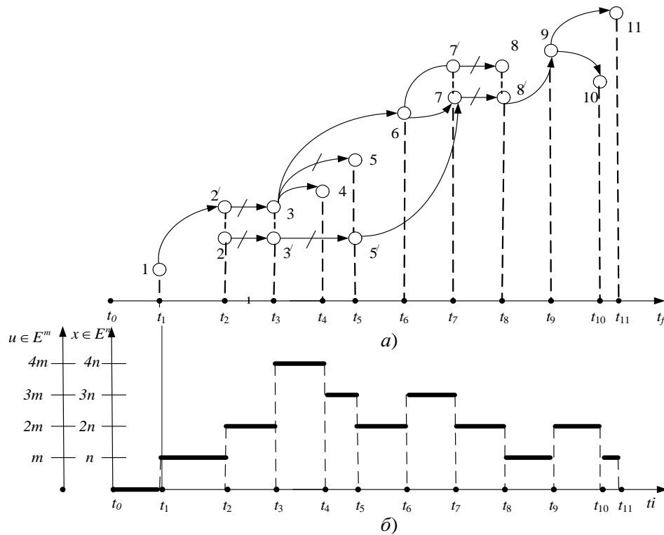
Рис. 6. Приклад структурної схеми розгалуженої траєкторії: а)- послідовність структурних перетворень в часі; б)- зміна розміру вектору стану і вектору керування розривної системи; t_i - моменти часу структурних перетворень СДС; стрілки умовно показують напрямок руху підсистем і блоків СДС
