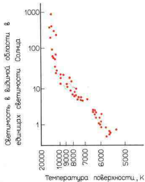
Рис. 2.7. Диаграмма Г-Р для звездного скопления Плеяды .
