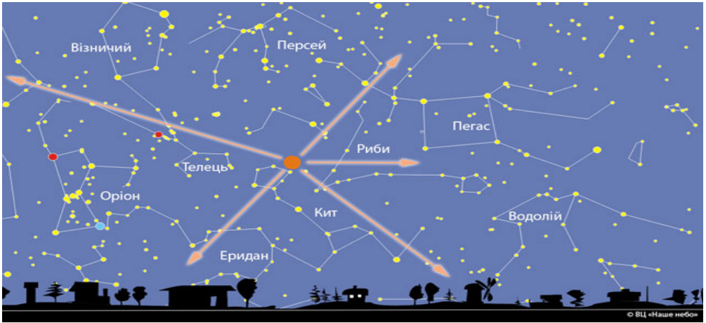
Положення радіанта метеорного потоку Цетиди (північно-східна ділянка зоряного неба).
