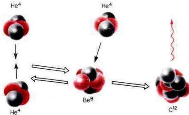
Рис. 3.4. Превращение гелия в углерод. Два ядра гелия сливаются с образованием чрезвычайно радиоактивного ядра бериллия, которое очень скоро снова распадется на два ядра гелия. Ядро изотопа бериллия превращается в ядро углерода (с испусканием кванта света) только в том случае, если за короткое время жизни изотопа \text{Be}^8 произойдет его столкновение с еще одним ядром гелия.
