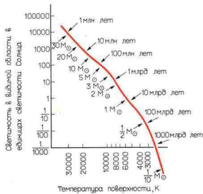
Рис. 2.11. Главная последовательность на диаграмме Г-Р.
