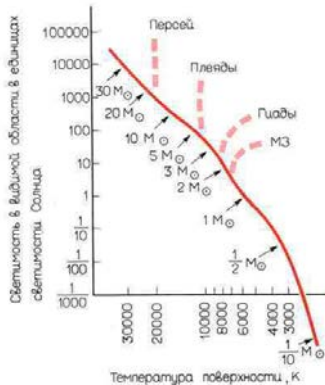
Рис. 2.10. Отклонение звезд различных скоплений от главной последовательности на диаграмме Г- Р (по данным Аллана Сандейджа).
