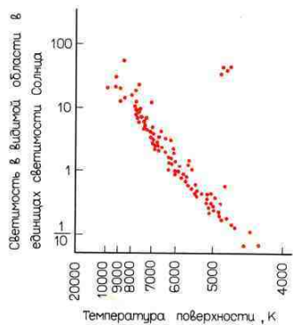
Рис. 2.8. Диаграмма Г- Р для звездного скопления Гиady . Если главная последовательность в Плеядax (см. рис. 2.1) простирается примерно до светимости в 1000 раз больше солнечной, то в Гиадах главная последовательность обрывается ниже 100 солнечных светимостей. Более яркие звезды главной последовательности отсутствуют. В то же время на диаграмме Г- Р этого скопления наблюдается группа красных гигантов.
