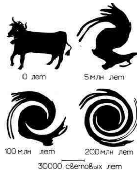
Рис. 12.5. Млечный Путь вращается не как твердое тело. Поэтому из произвольной начальной структуры через 100 миллионов лет образуется спиральный объект. К сожалению, спиральные рукава нашей Галактики не поддаются такому объяснению.
