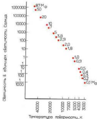
Рис. 4.3. Точками показаны данные для звезд с разной массой, полученные с помощью компьютерной модели. Все звезды состоят из богатой водородом смеси одинакового состава. На диаграмме Г-Р они образуют главную последовательность со всеми свойствами наблюдаемой главной последовательности. Массы звезд выражены в единицах массы Солнца M_{\odot} . Видно, что светимость звезд главной последовательности резко падает с уменьшением массы.
