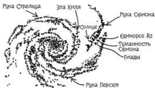
Галактика Млечный Путь
