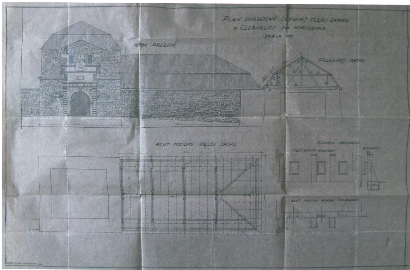
План-креслення відбудови замку. 1920-ті рр. Державний архів Львівської області
