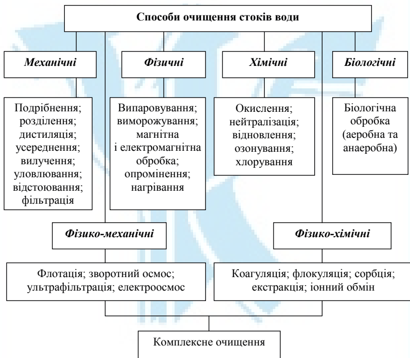
Рис. 6.12. Класифікація способів очищення стічних вод
