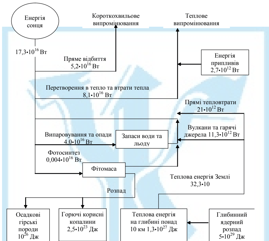
Рис. 2.7. Планетарний потік енергії (за Скіннером, 1989)
