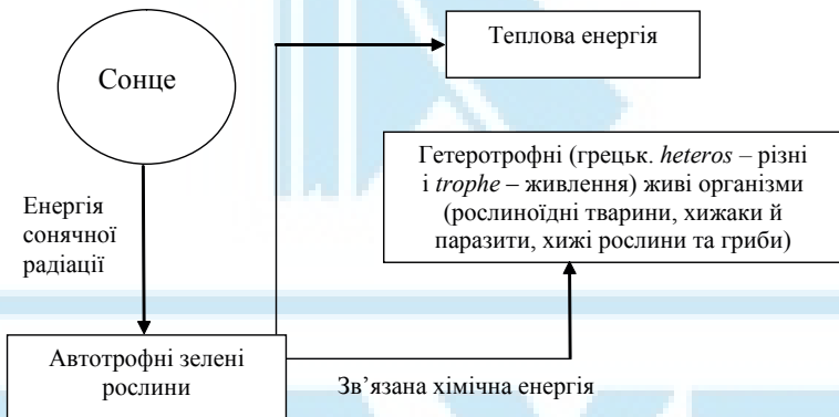
Рис. 2.6. Основні напрями потоку енергії на Земній кулі
